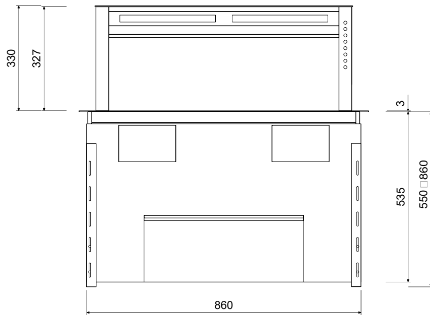
正面図
