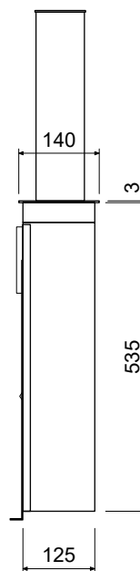
側面図
