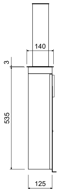
側面図
