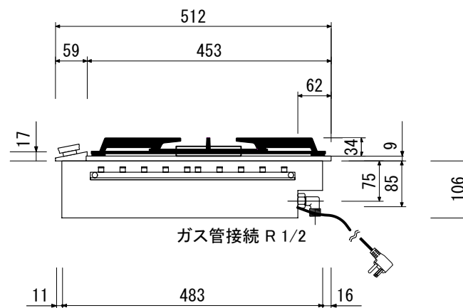
側面図
