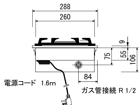
背面図
