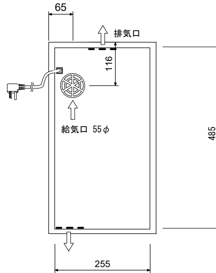
底面図
