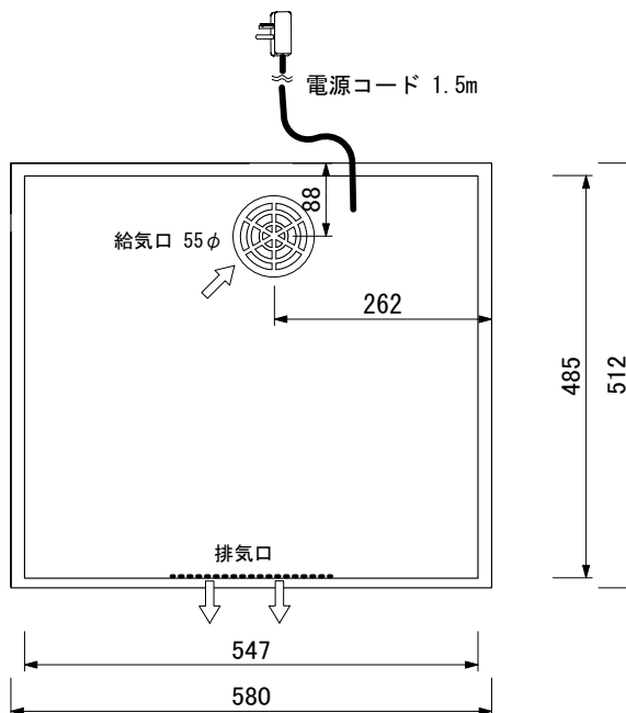
底面図
