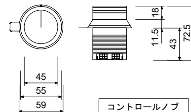
コントロールノブ
