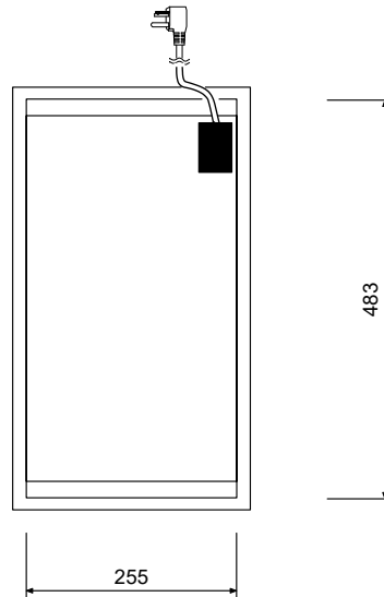
底面図
