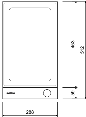
上面図
