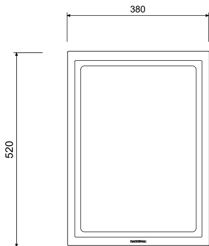
上面図
