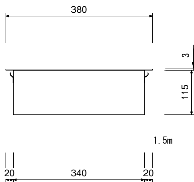
正面図
