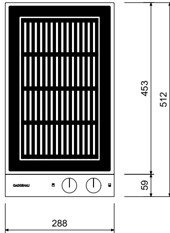
上面図
