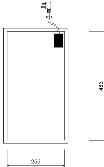
底面図
