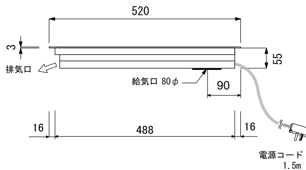
側面図
