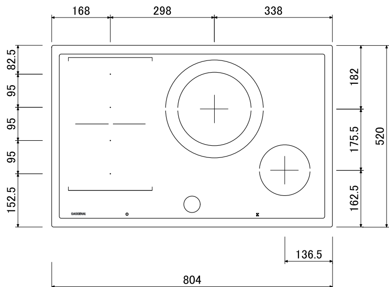
上面図
