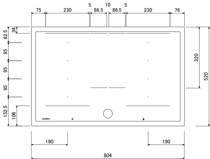
上面図
