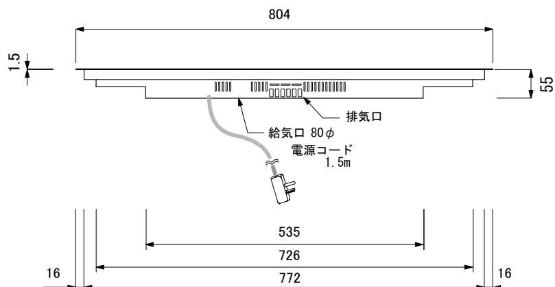
正面図
