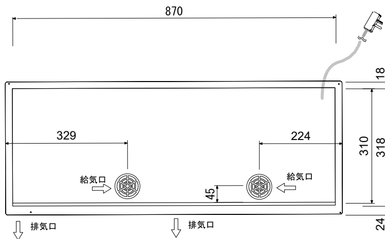
底面図
