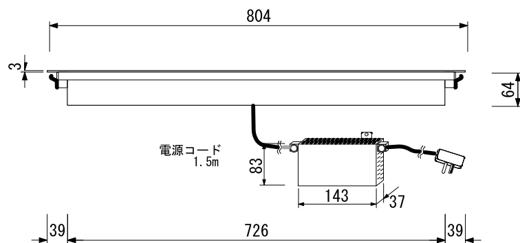
正面図
