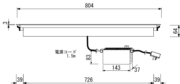
正面図
